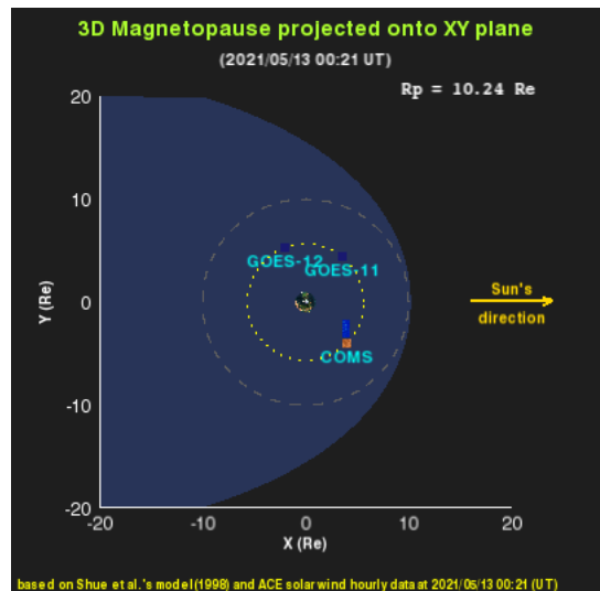
지구자기권계면의 위치
