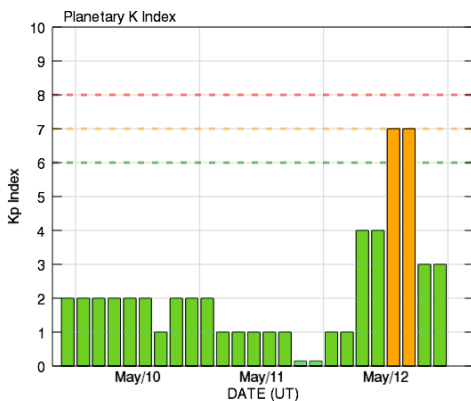
지구자기장 교란지수
