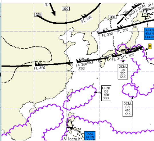
공역예보(SIGWX) 10.26. 15:00KST
