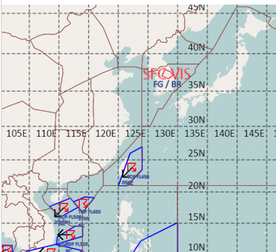
공역경보(SIGMET) 10.26. 08:00KST
