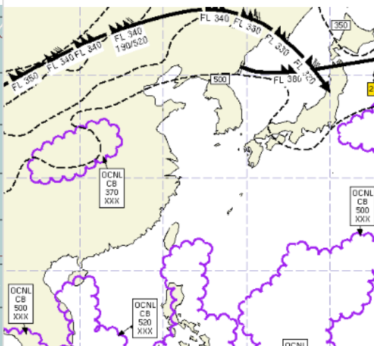
공역예보(SIGWX) 10.17. 03:00KST
