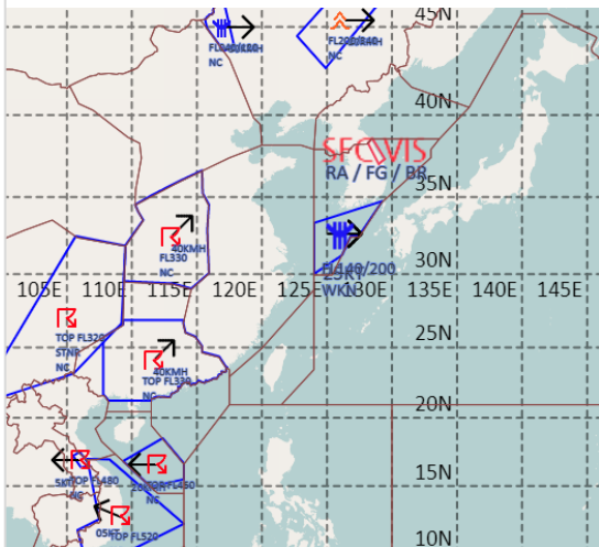
공역경보(SIGMET) 10.16. 15:00KST
