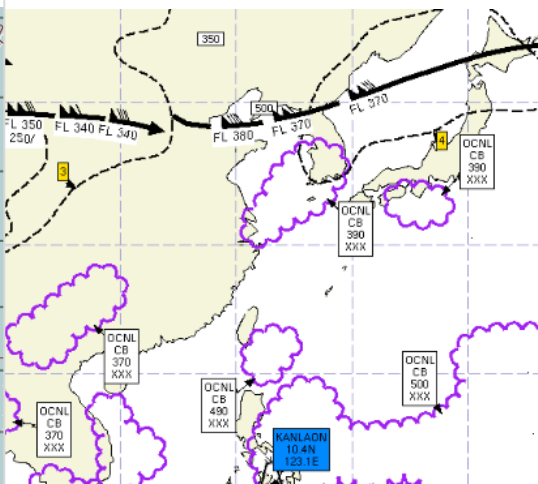
공역예보(SIGWX) 10.16. 03:00KST
