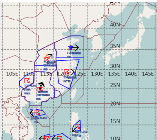
공역경보(SIGMET) 10.15. 15:00KST
