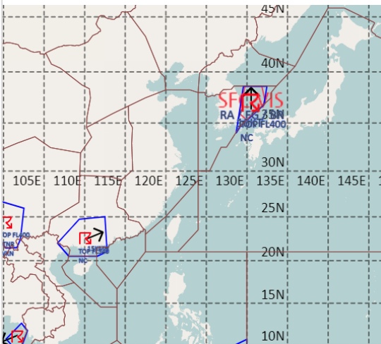
공역경보(SIGMET) 07.14. 08:00KST
