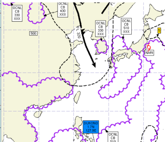
공역예보(SIGWX) 07.14. 15:00KST
