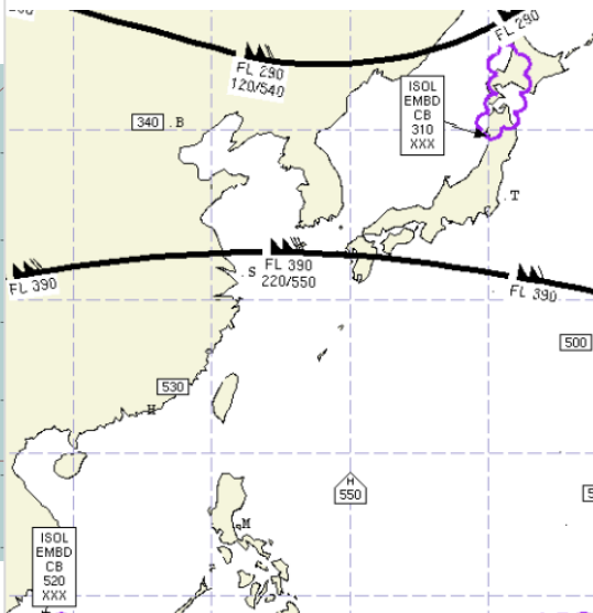
공역예보(SIGWX) 12.09. 15:00KST
