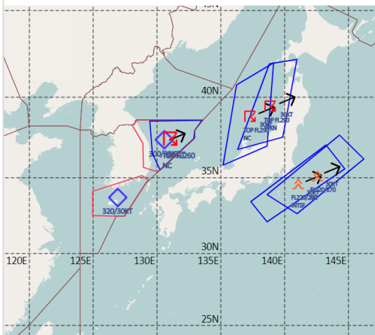
공역경보(SIGMET) 12.07. 08:00KST
