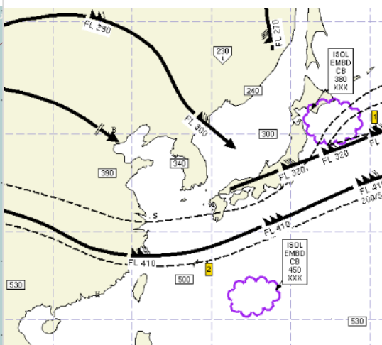
공역예보(SIGWX) 12.07. 15:00KST
