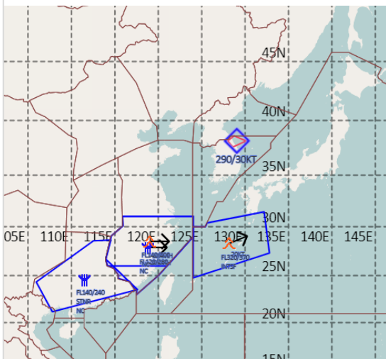
공역경보(SIGMET) 12.04. 15:00KST
