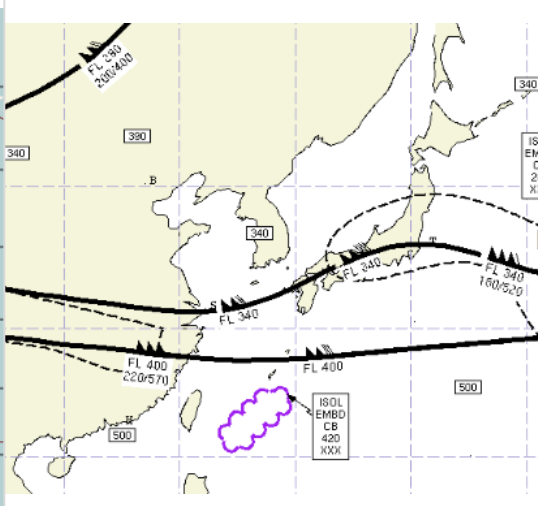
공역예보(SIGWX) 12.05. 03:00KST
