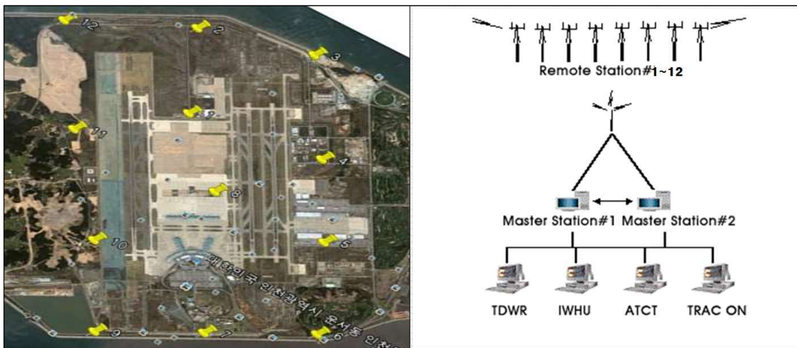
[그림 4] 인천국제공항의 저층급변풍경고장비 구성 현황
