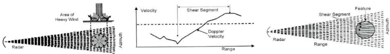
[그림 7] TDWR 급변풍(Wind shear) 및 마이크로버스트(Microburst) 발생 패턴 분석
