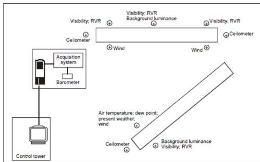
[그림 1] 항공기상관측 시스템 구성도(ICAO Doc 9837, Figure 11-1)
