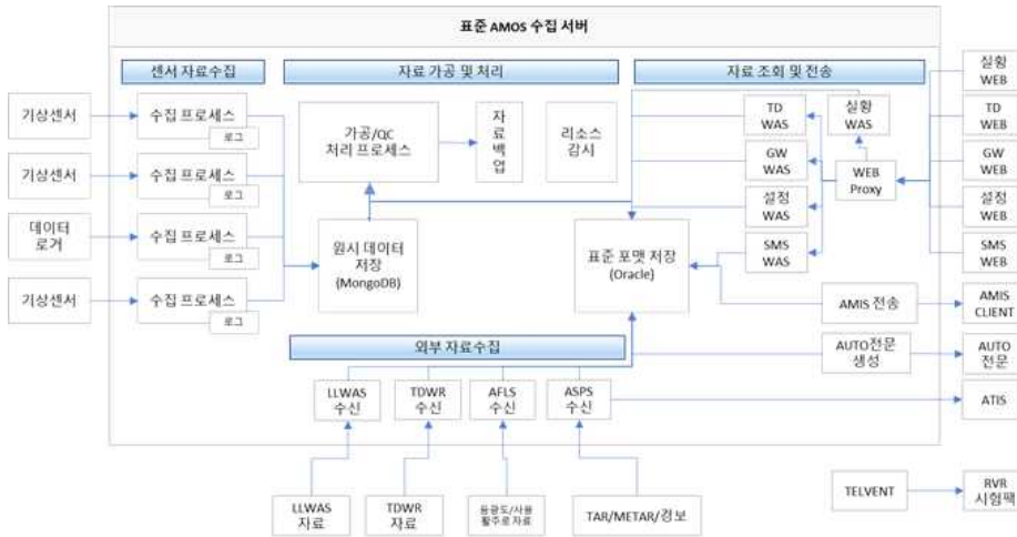
[그림 2] AMOS 관측자료 수집·처리·표출 흐름도
