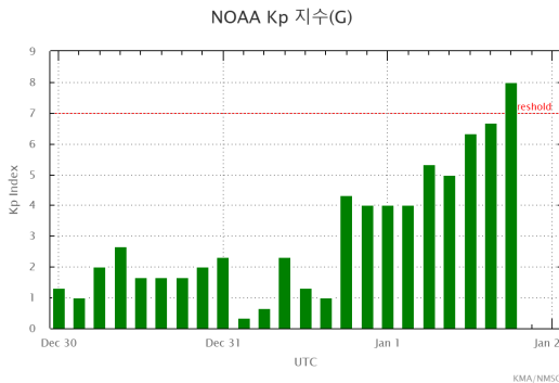
지구자기장 교란지수
