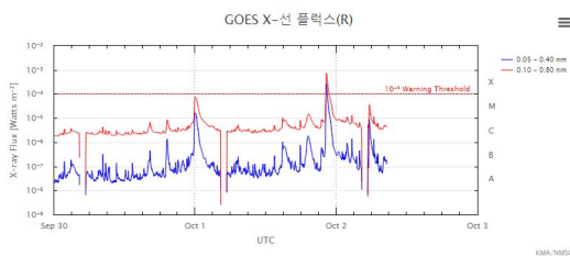
태양 엑스선 플럭스
