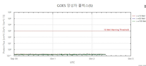
태양 고에너지 입자 플럭스
