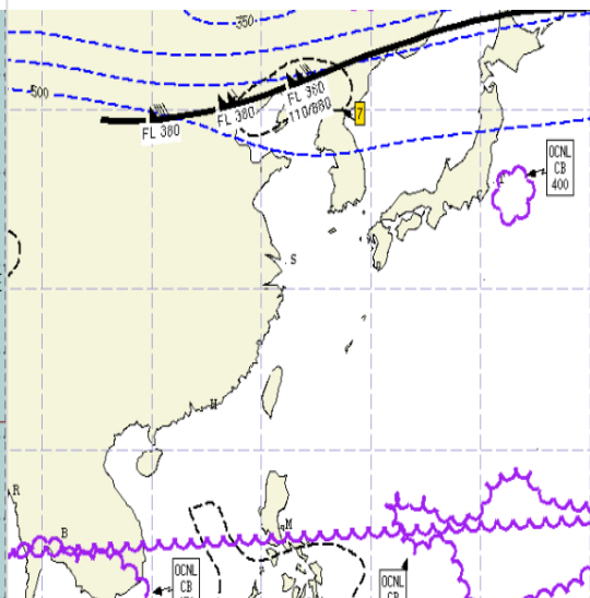
공역예보(SIGWX) 09.13. 03:00KST
