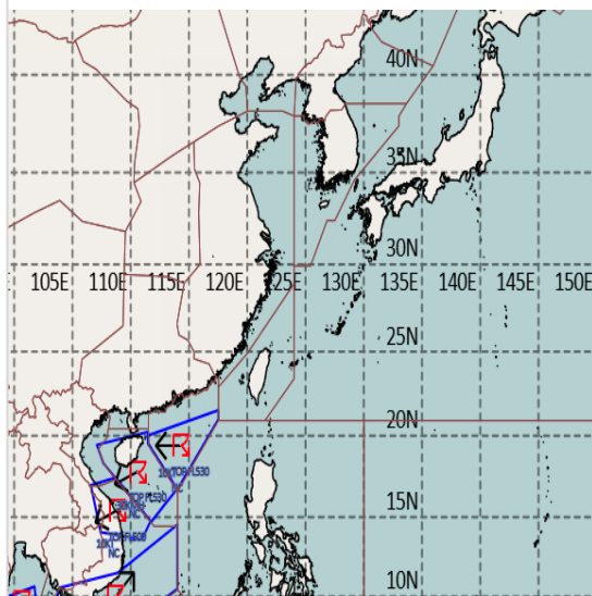
공역경보(SIGMET) 09.12. 15:00KST
