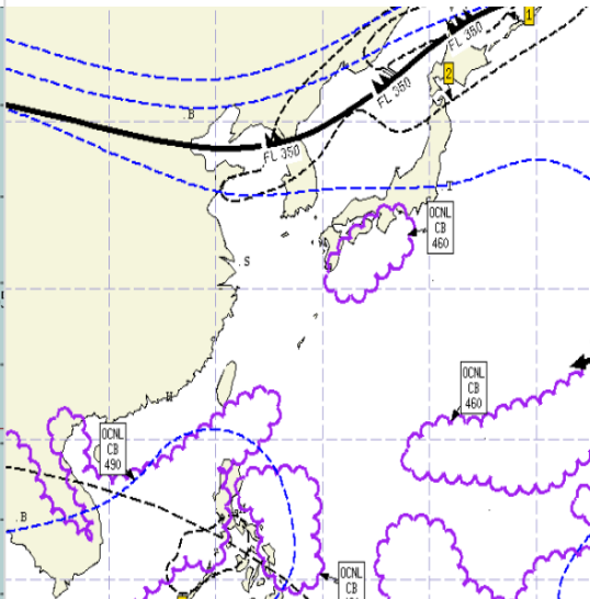
공역예보(SIGWX) 09.11. 03:00KST
