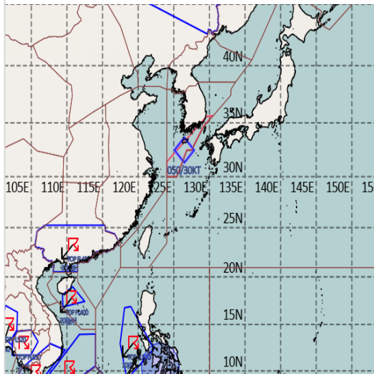
공역경보(SIGMET) 09.10. 15:00KST
