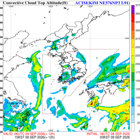
공역예보(SIGWX) 09.09. 15:00KST
