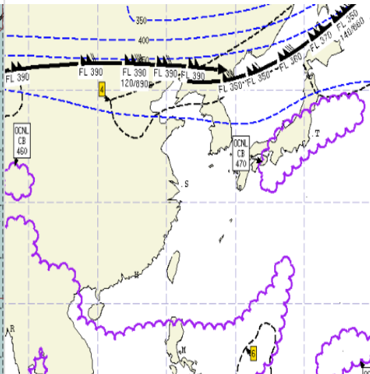
공역예보(SIGWX) 09.09. 15:00KST
