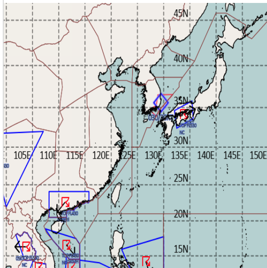
공역경보(SIGMET) 09.09. 08:00KST
