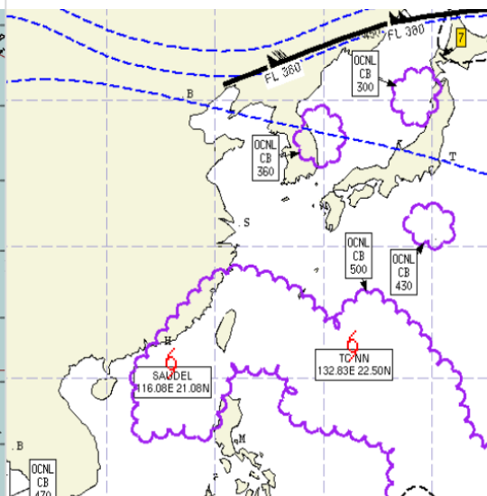
공역예보(SIGWX) 09.02. 03:00KST
