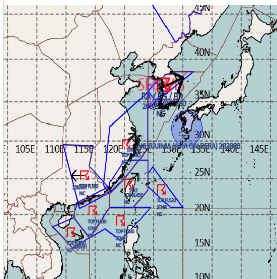
공역경보(SIGMET) 09.01. 15:00KST
