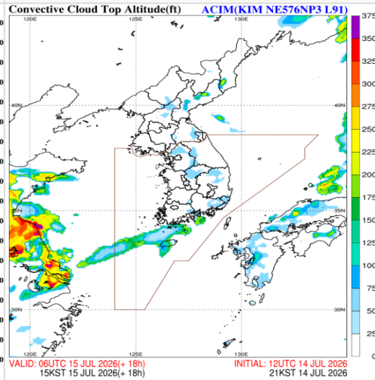
공역예보(SIGWX) 07.15. 15:00KST
