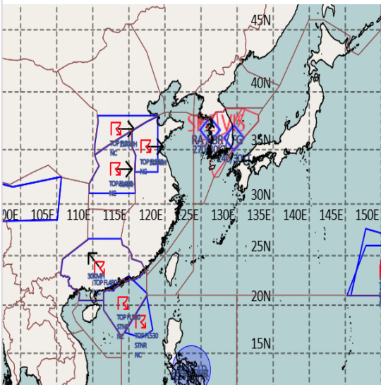
공역경보(SIGMET) 07.15. 08:00KST
