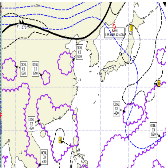
공역예보(SIGWX) 07.15. 15:00KST
