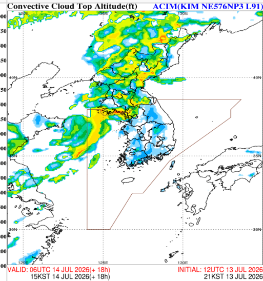
공역예보(SIGWX) 07.14. 15:00KST
