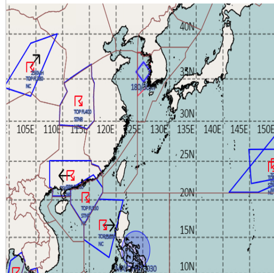
공역경보(SIGMET) 07.14. 08:00KST
