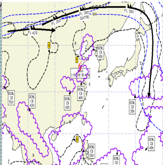
공역예보(SIGWX) 07.14. 03:00KST
