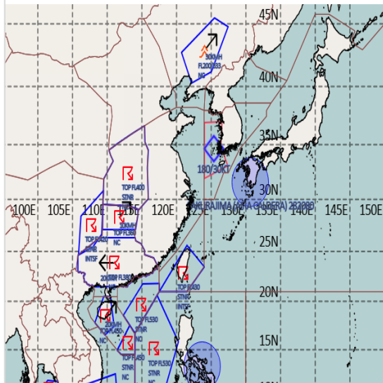
공역경보(SIGMET) 07.13. 15:00KST
