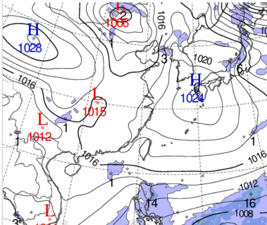
공역경보(SIGMET) 01.14. 08:00KST
