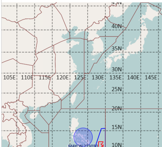
공역경보(SIGMET) 01.14. 08:00KST
