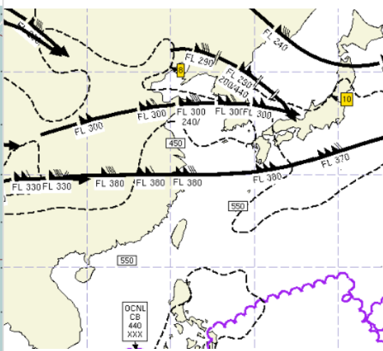
공역예보(SIGWX) 01.14. 15:00KST
