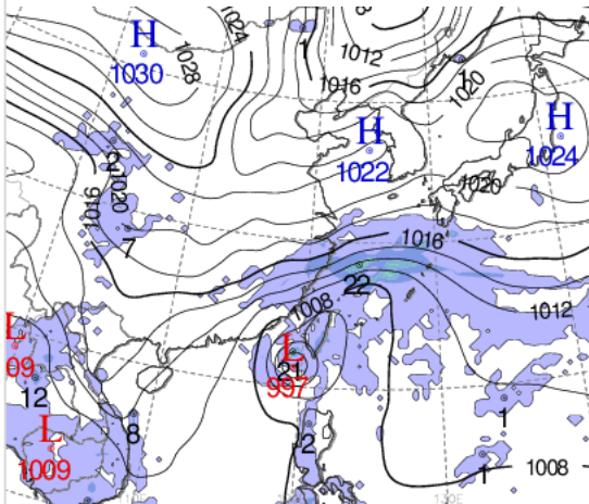
공역경보(SIGMET) 11.12. 08:00KST
