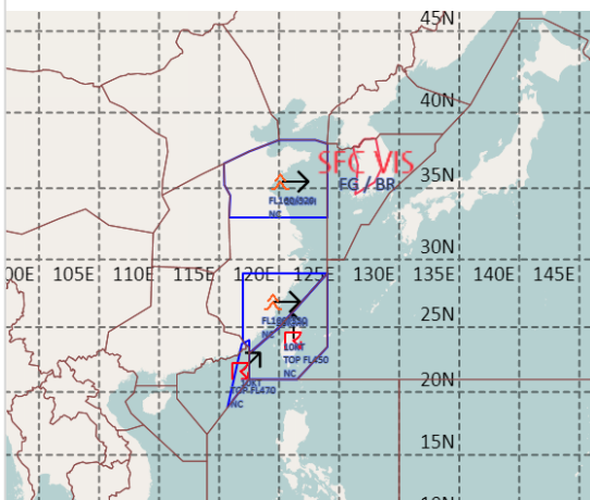
공역경보(SIGMET) 11.12. 08:00KST
