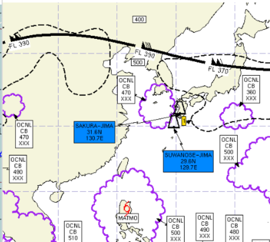
공역예보(SIGWX) 10.03. 15:00KST
