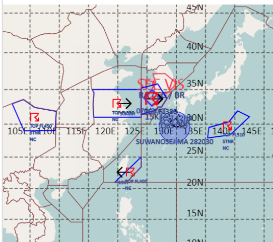
공역경보(SIGMET) 10.03. 08:00KST
