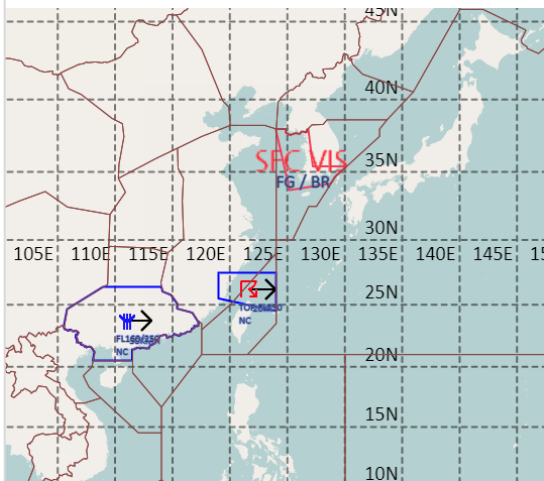
공역경보(SIGMET) 04.18. 08:00KST
