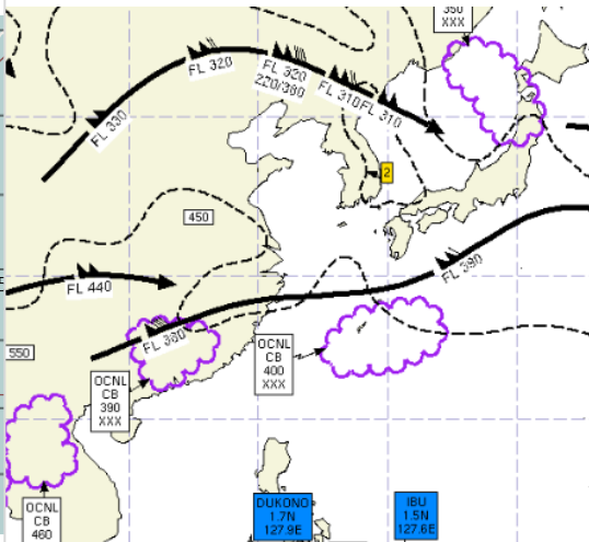
공역예보(SIGWX) 04.18. 15:00KST
