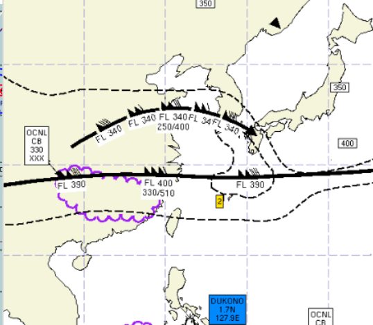
공역예보(SIGWX) 04.09. 15:00KST
