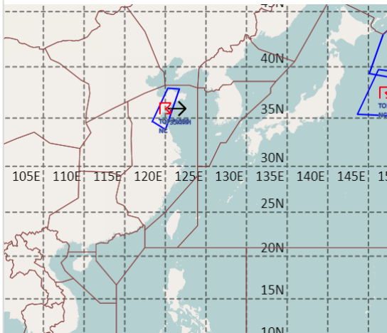
공역경보(SIGMET) 04.09. 08:00KST
