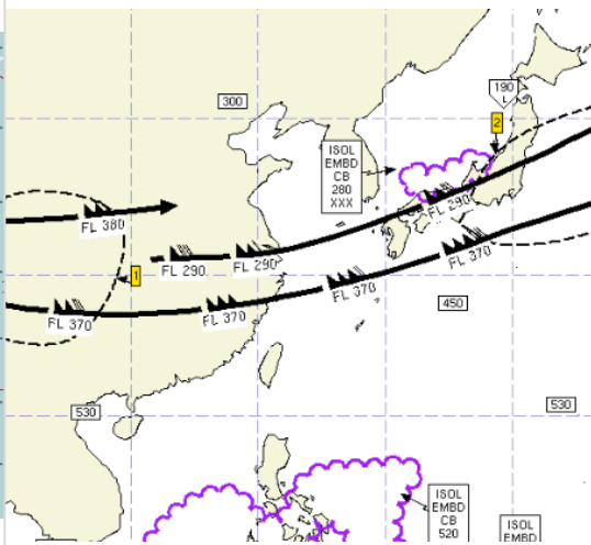
공역예보(SIGWX) 01.10. 03:00KST
