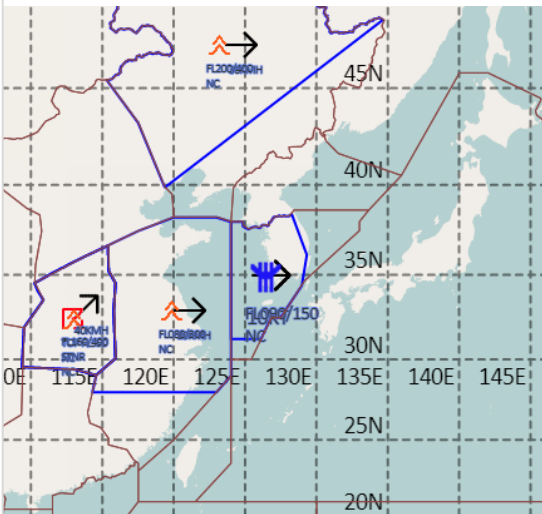
공역경보(SIGMET) 02.18. 15:00KST
