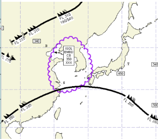
공역예보(SIGWX) 02.19. 03:00KST
