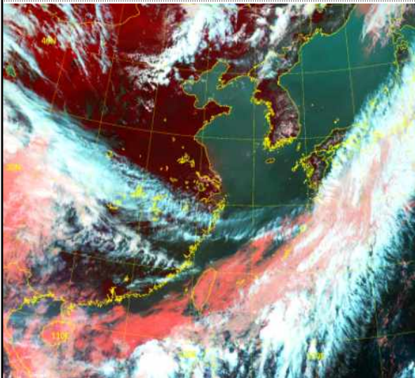
위성영상 (5. 17. 15:00KST)
