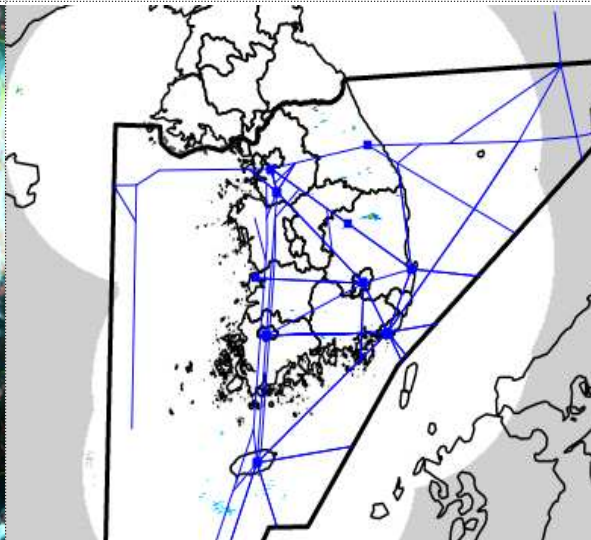
레이더영상 (5. 17. 15:00KST)
